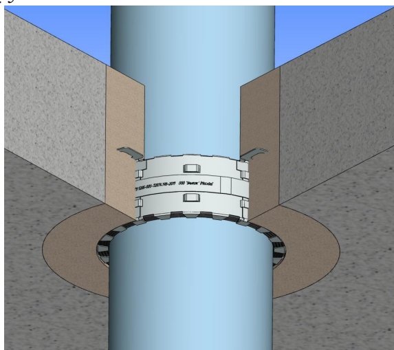
Установка противопожарных муфт Феникс ППМ при проходе вертикального трубопровода через перекрытие из железобетона с полным заглублением в цементный раствор (только для труб до 63мм)
