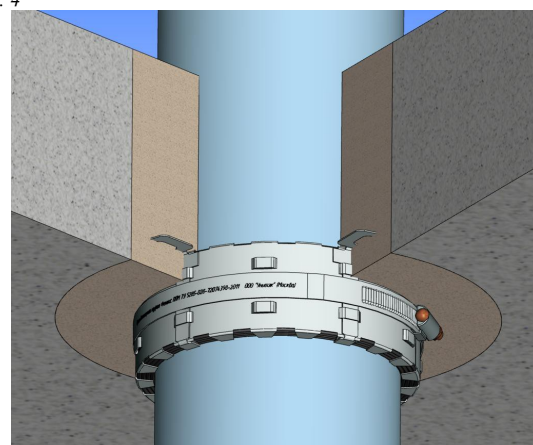
Установка противопожарных муфт Феникс ППМ при проходе вертикального трубопровода через перекрытие из железобетона – заглубленная на 10-15 мм установка в цементный раствор
